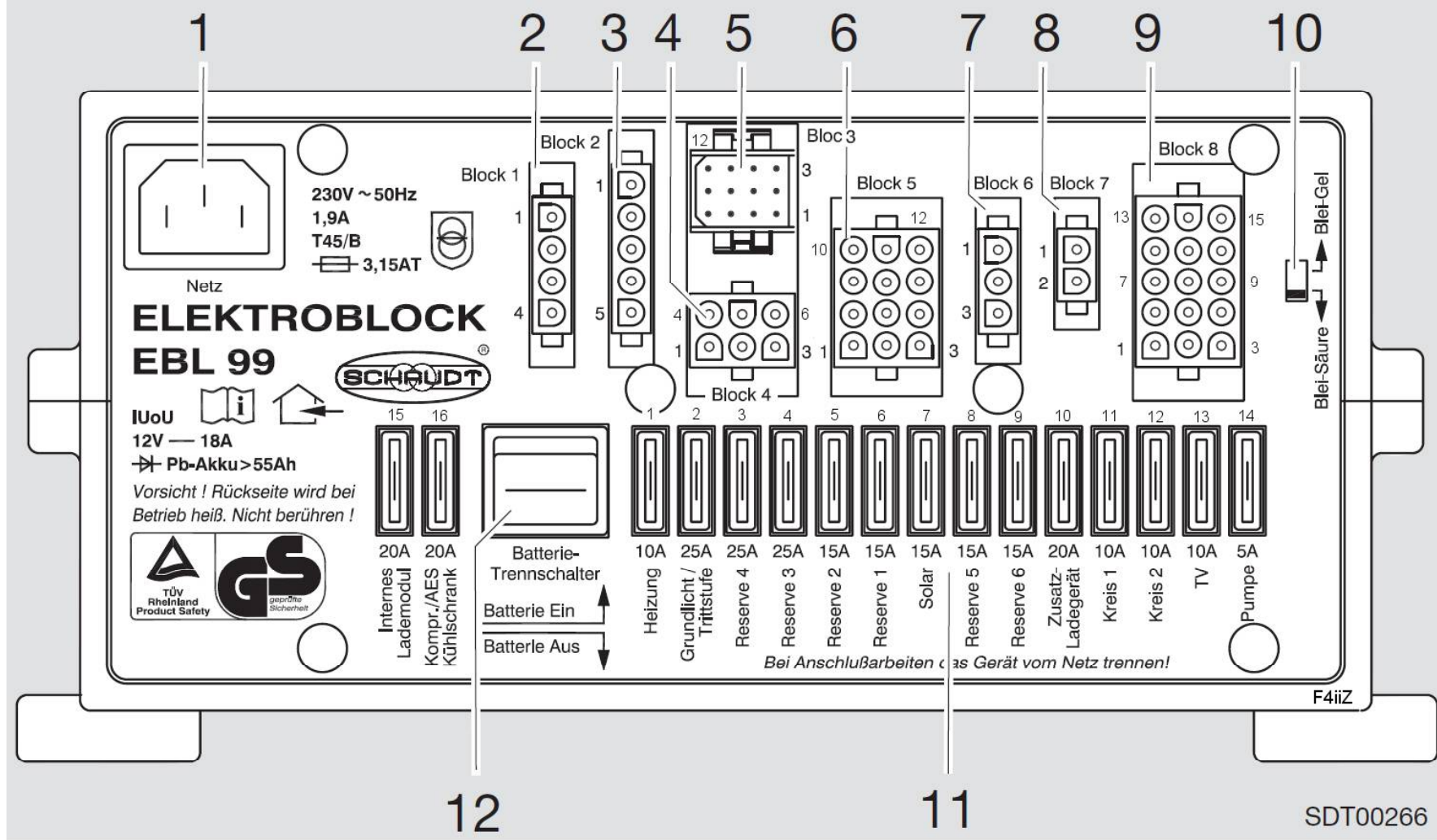
Fig. 1 Vue frontale du bloc électrique EBL 99 G
